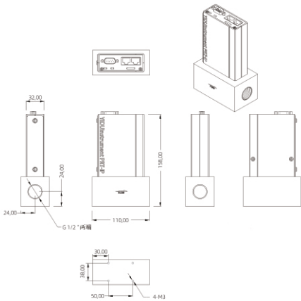
图:外形尺寸图3
