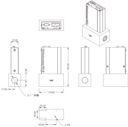
图:外形尺寸图4
