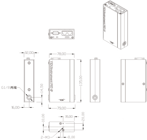
图:外形尺寸图1
