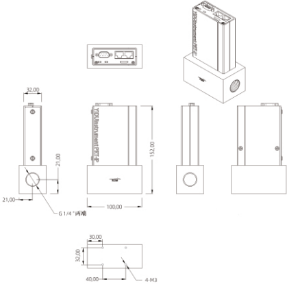
图:外形尺寸图2
